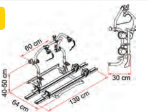
Carry-Bike Pro C E-Bike Zur Befestigung unterhalb des Fensters 440680 1 438,- 440681* 1 439,-
