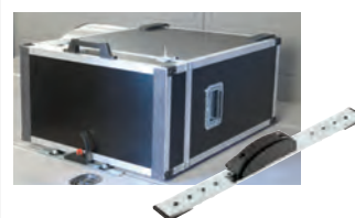
Adapter • Beliebig an Schiene einsetzbar • 1-Hebel-Handhabung (Stahl) zur Befestigung von Schränken, Wänden, Behältern Maße: 400 x 35 x 44 mm Bohrungen M8, 1500 daN 44330 1 169,-
