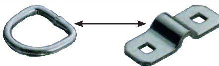
Zurrplatte, Belastbarkeit: 200 daN, Höhe: 11 mm 44316 1 3,20 Lasche für D-Ring, Lochabstand 45 mm 44315 1 2,99
