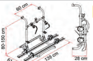
Carry-Bike Bike Pro E für E-Bike Für die Reisemobil Rückwand 440216 1 438,95 440217* 1 439,-
