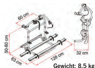
Carry-Bike PRO M Zur Befestigung unterhalb des Fensters 440213 1 279,-
