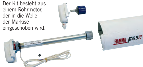
Rohrmotor F 65
