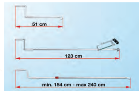
Rändel
